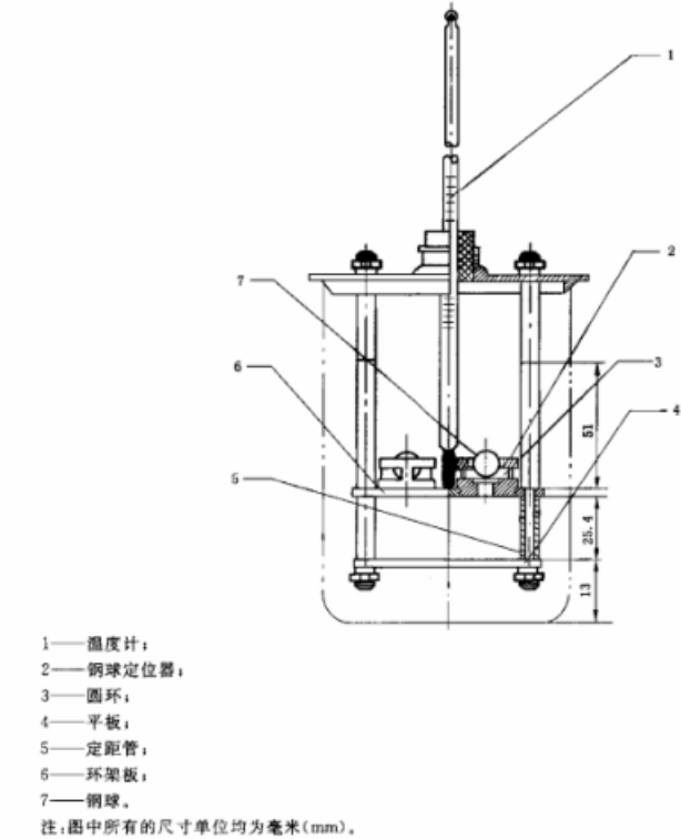
图 1 软化点测定器
