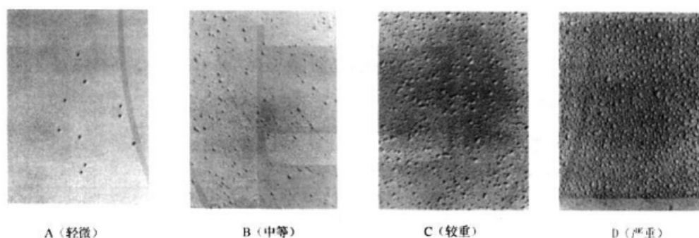
图 3 盐雾试验后样板表面漆膜起泡图例
