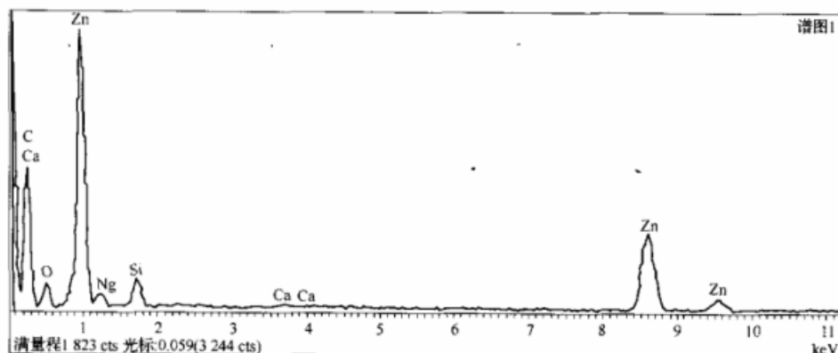
图2 富锌涂料漆膜扫描电镜谱图
